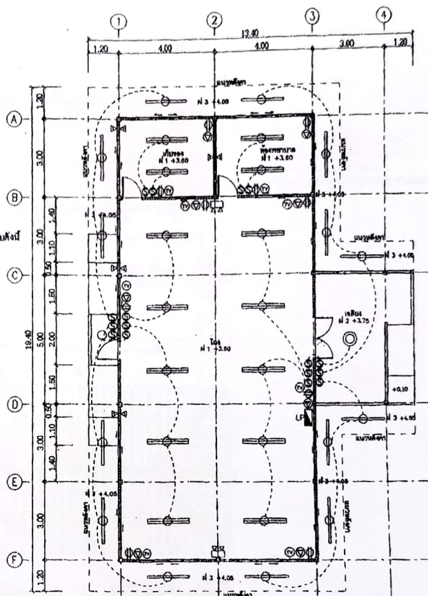
แปลนระบบไฟฟ้า มาตรฐาน 1:100
