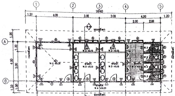
แปลนพื้นที่ 1 มาตราส่วน 1:100
